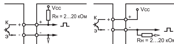
Схемы включения транзисторного выхода
